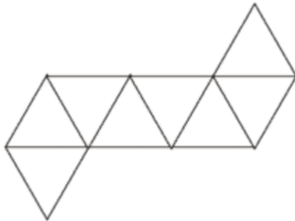
正8面体の展開図 11種類
