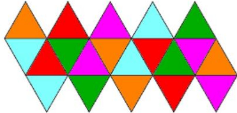
正20面体の展開図 43,380 種類
